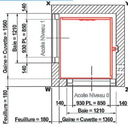
Service équerre - Gaine béton
