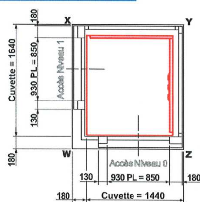
Service équerre - Pylone tolé ou vitré
