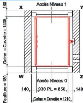
Service équerre - Gaine béton
