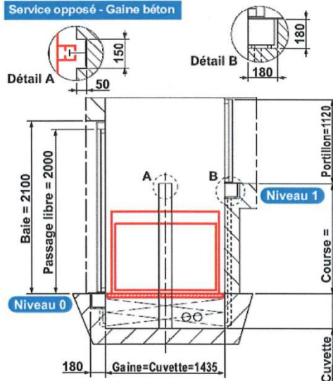
Service opposé - Gaine béton
