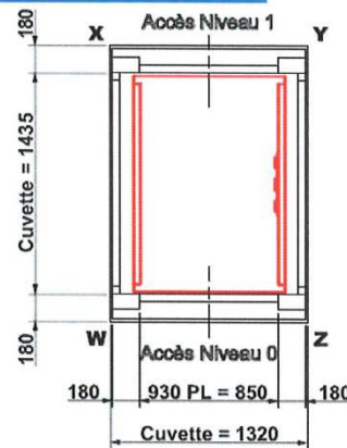
Service équerre - Pylone tolé ou vitré
